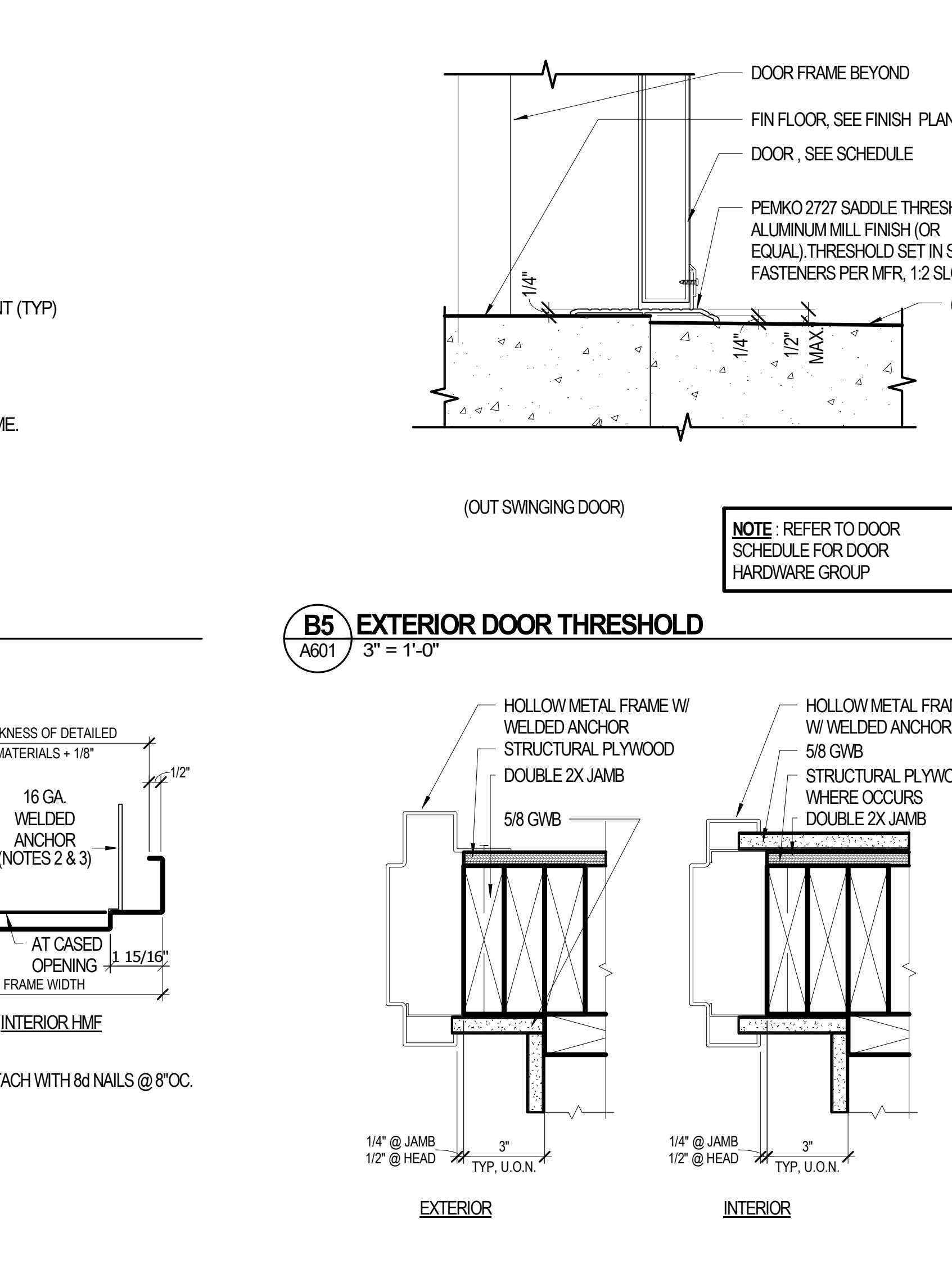
A5 HOLLOW METAL FRAME - JAMB A601 3" = 1'-0"
