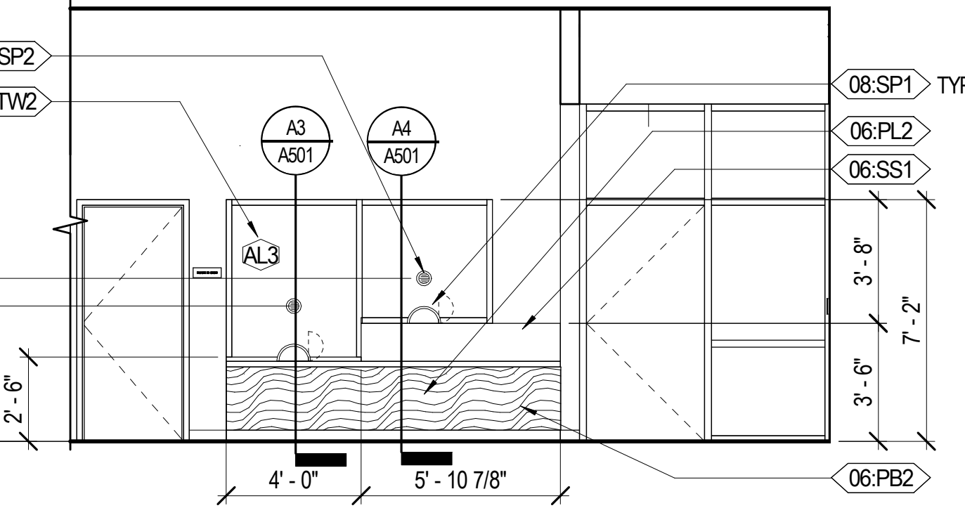
E4 CORRIDOR 106 A251 1/4" = 1'-0"
