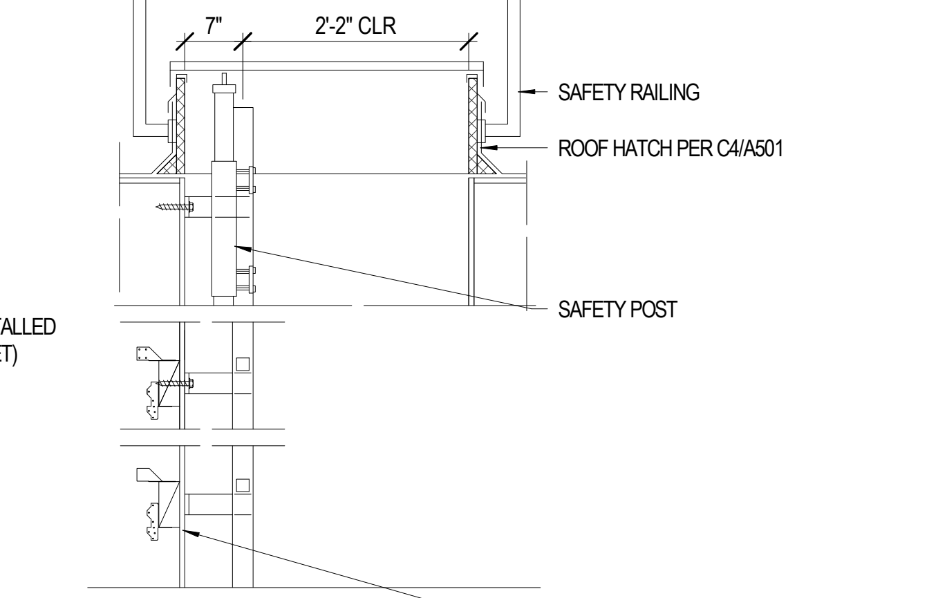
C4 ROOF HATCH A501 3" = 1'-0"
