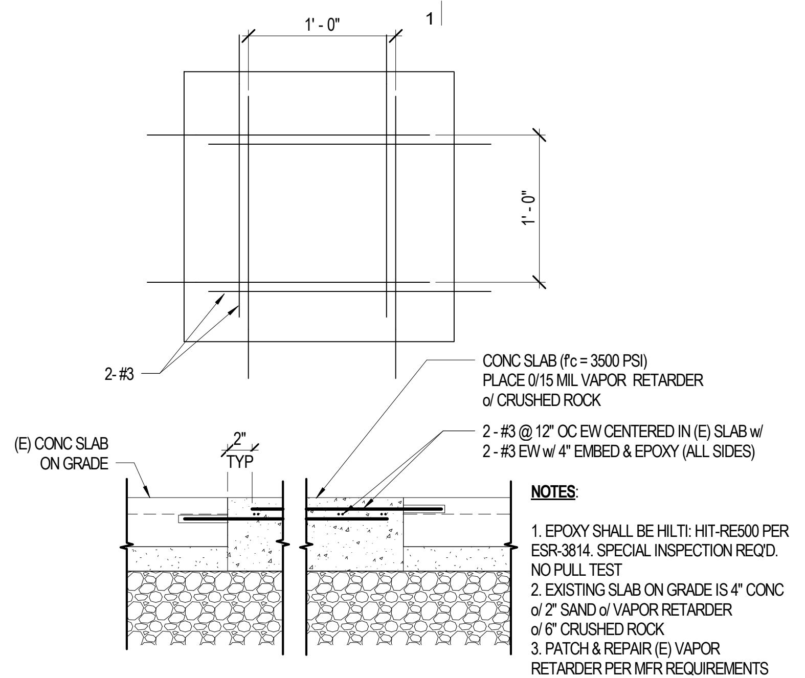
D1 (E) SLAB REPAIR A501 1 1/2" = 1'-0"
