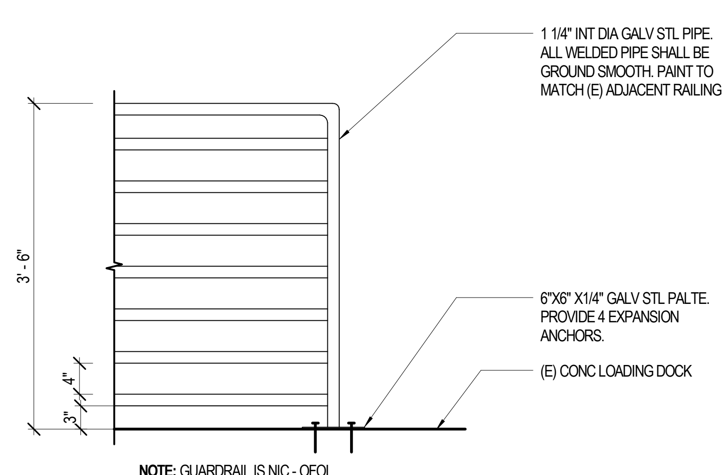
A2 #3 - OFOI A102 1" = 1'-0"
