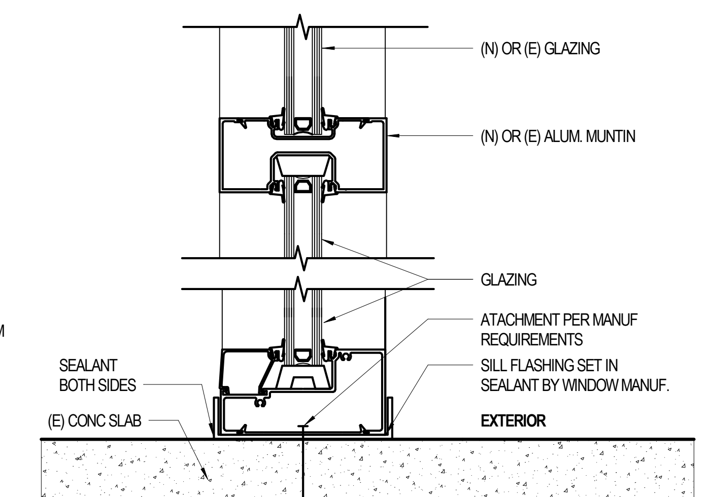
A5 EXTERIOR STOREFRONT SILL A602 3" = 1'-0"
