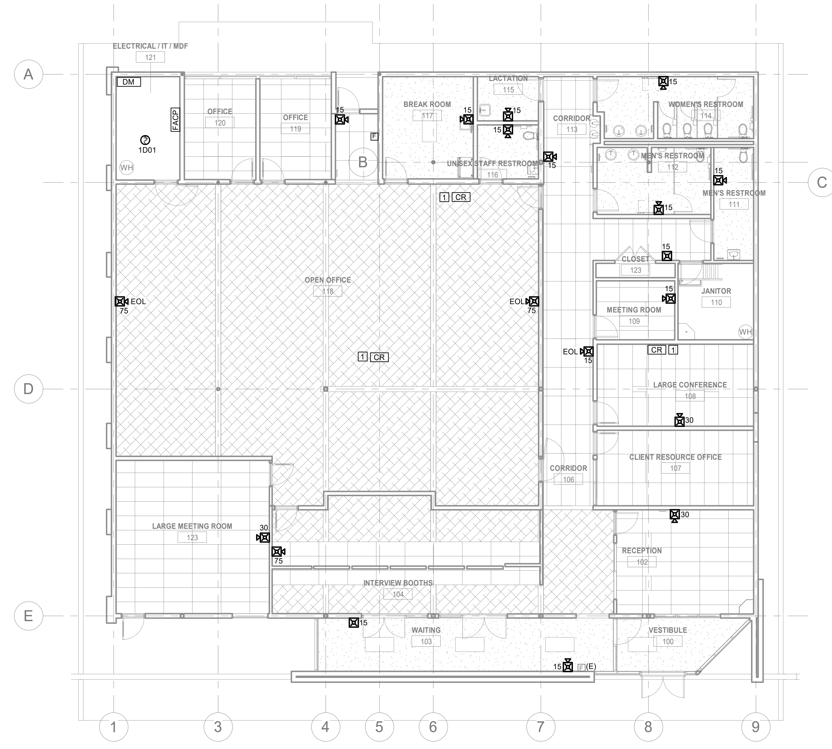
1 FIRE ALARM PLAN - LEVEL 01 SCALE: 1/8" = 1'-0"
