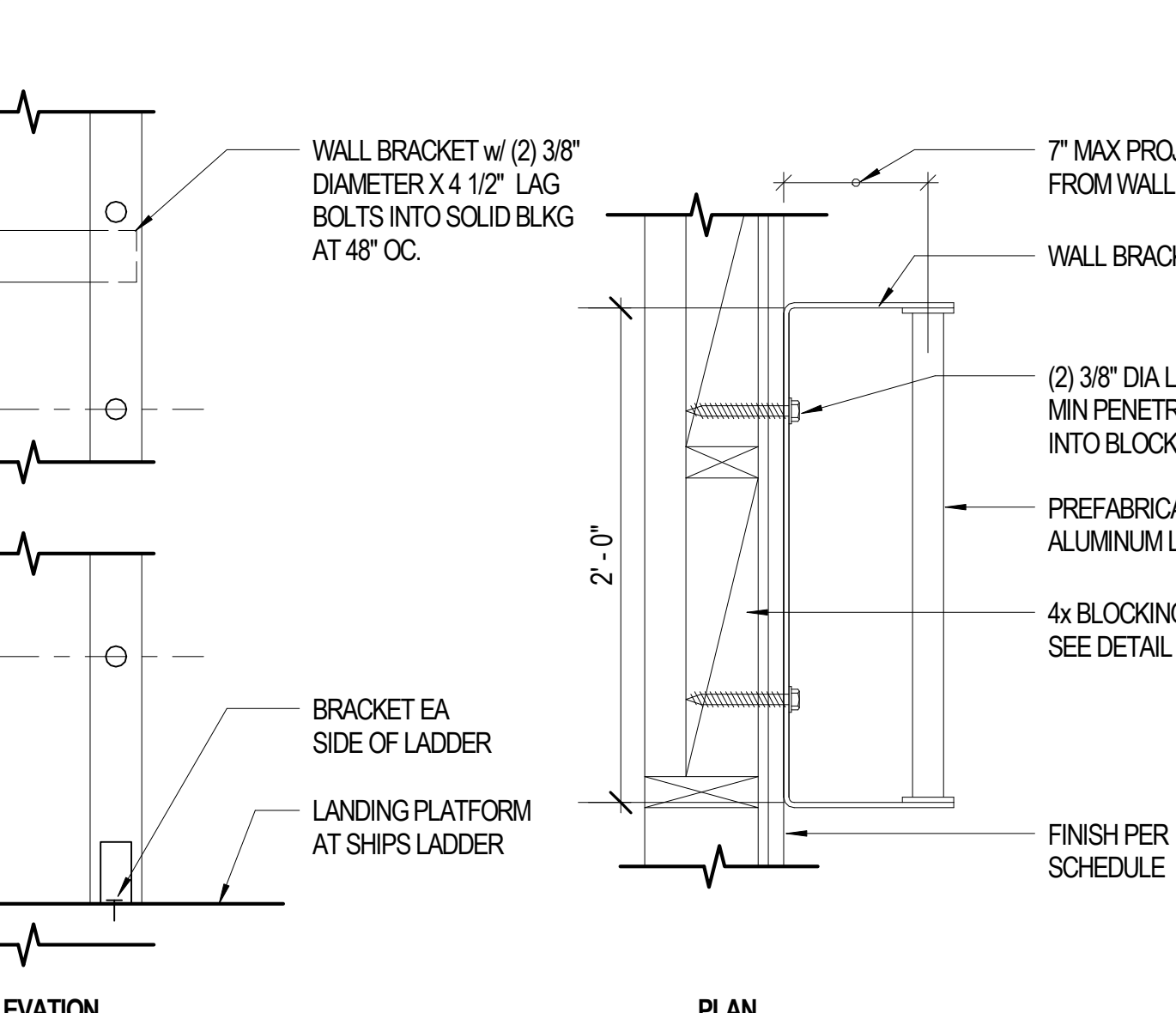
A6 INTERIOR ALUM LADDER A501 1 1/2" = 1'-0"
