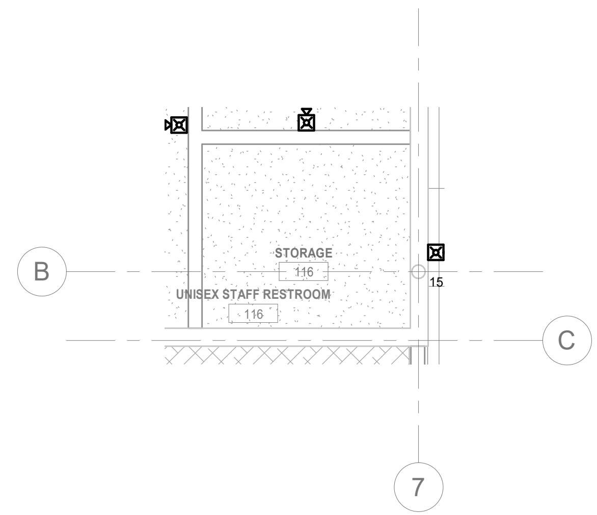
3 FIRE ALARM PLAN - ALT#4 SCALE: 1/4" = 1'-0"
