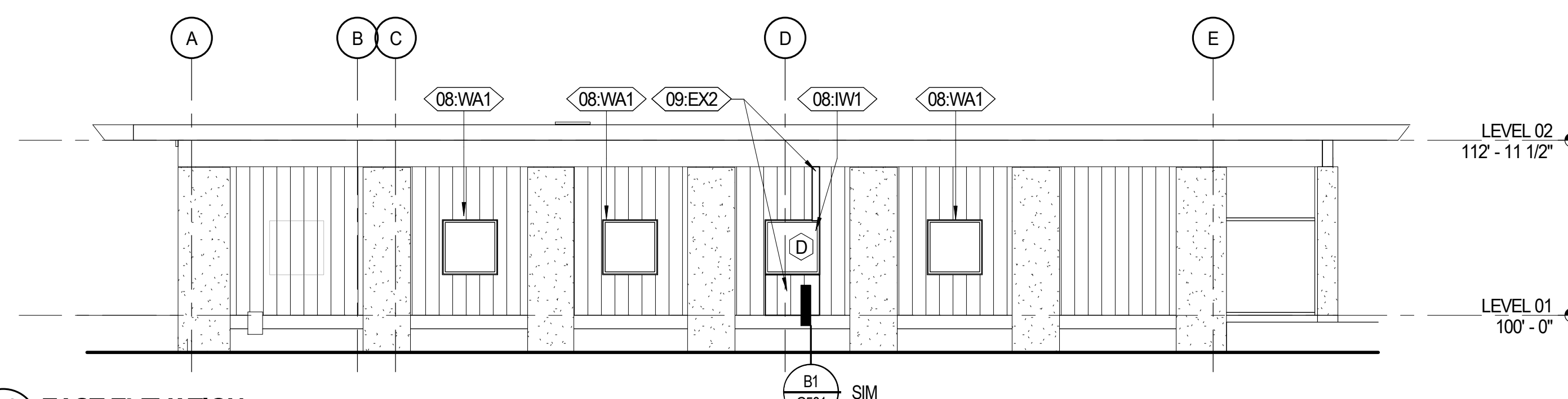
A3 EAST ELEVATION A201 1/8" = 1'-0"
