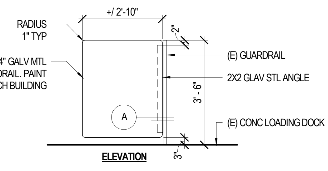
6 GUARDRAIL SOUTH ENTRANCE - OFOI G501 1/2" = 1'-0"
