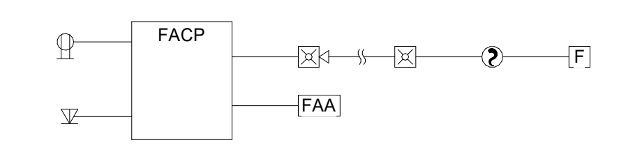
4 Fire Alarm Riser Diagram SCALE: 12" = 1'-0"
