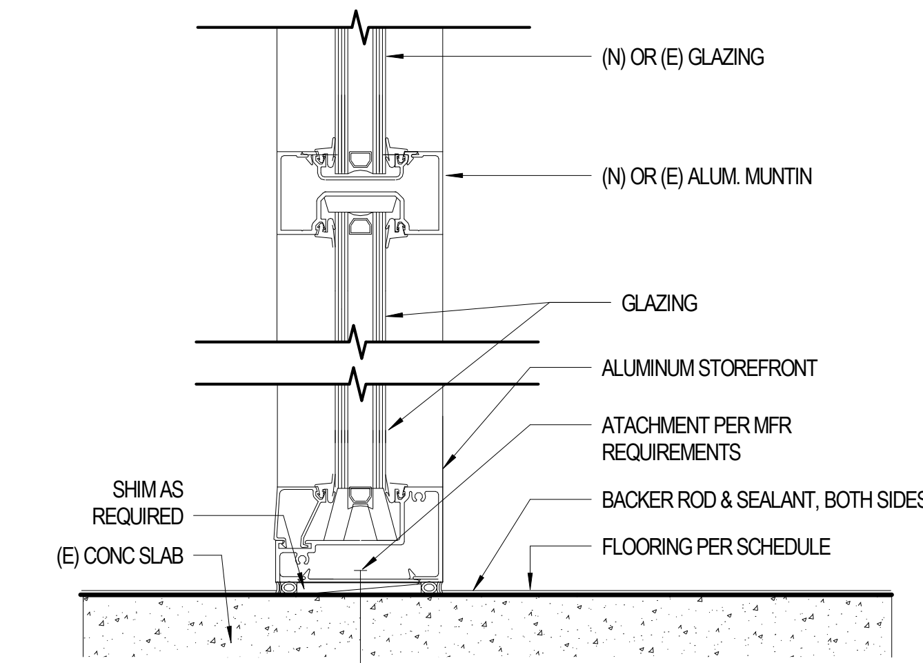
B4 STOREFRONT SILL A602 3" = 1'-0"
