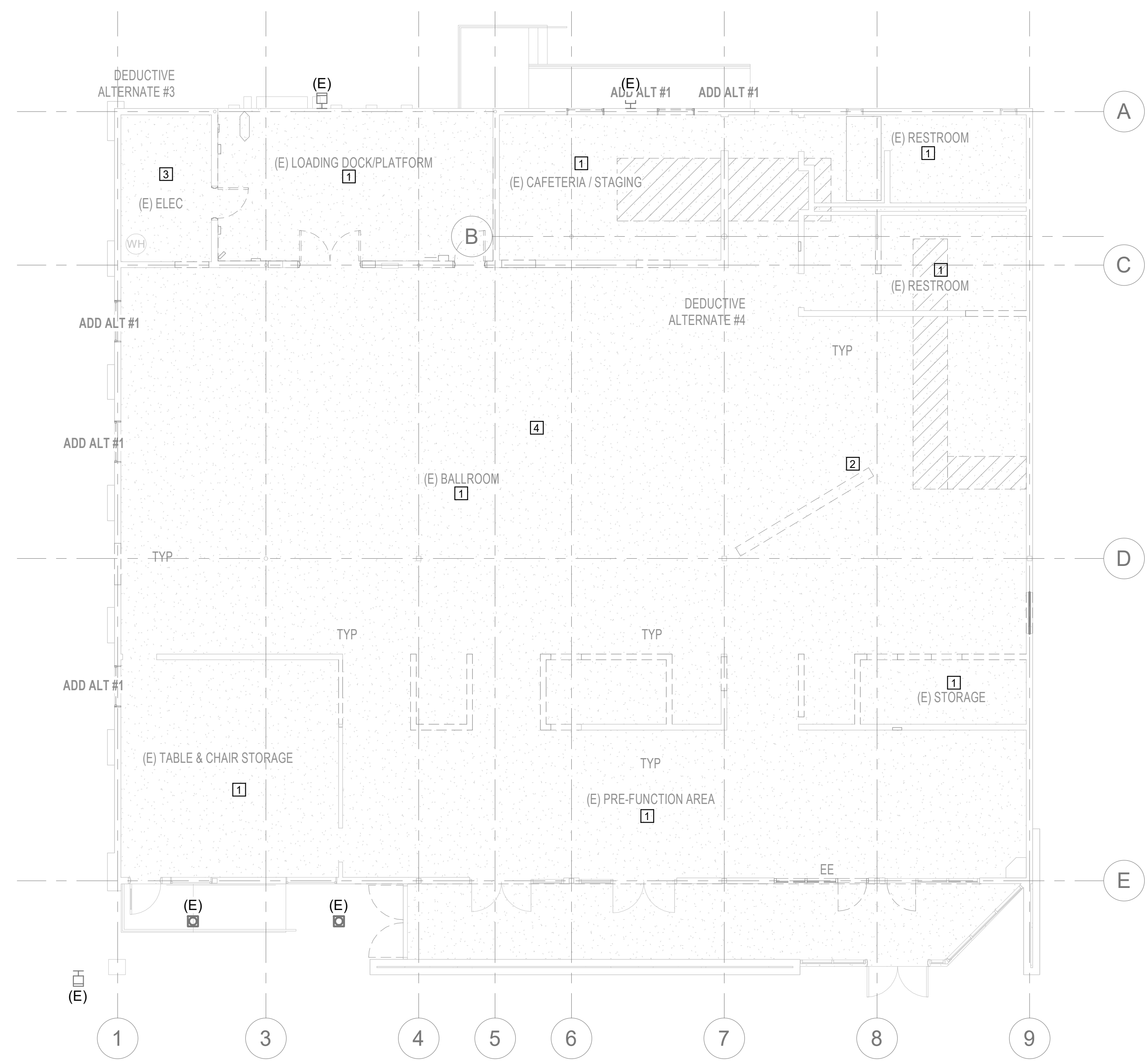
1 DEMO PLAN - LEVEL 01 SCALE: 1/8" = 1'-0"
