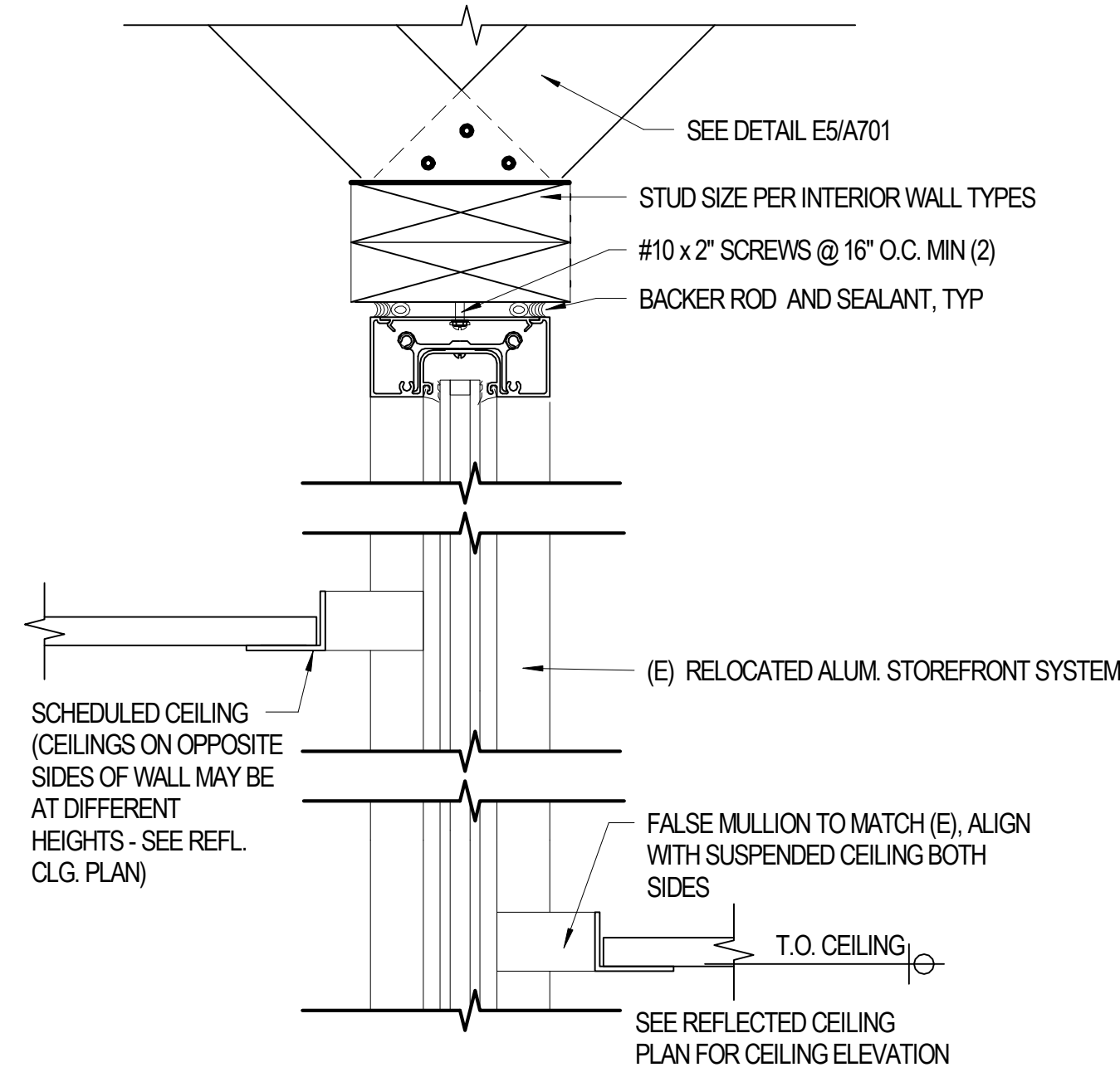
D3 INTERIOR STOREFRONT A602 3" = 1'-0"
