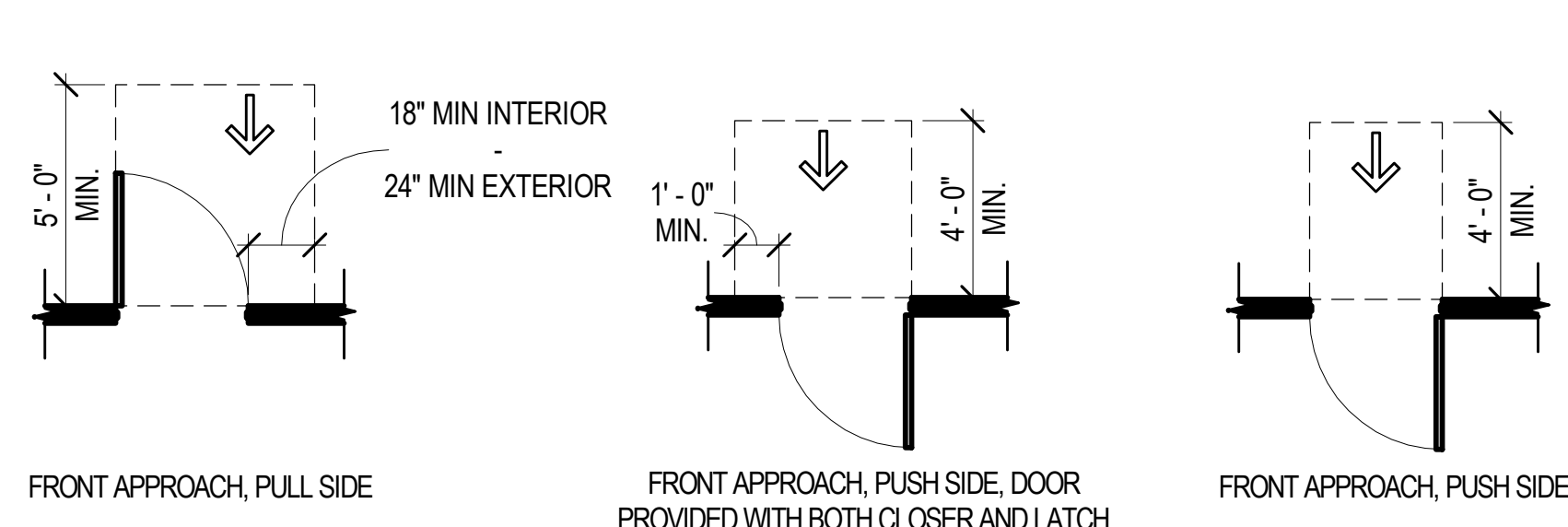
E2 ADA DOOR CLEARANCES G701 1/4" = 1'-0"
