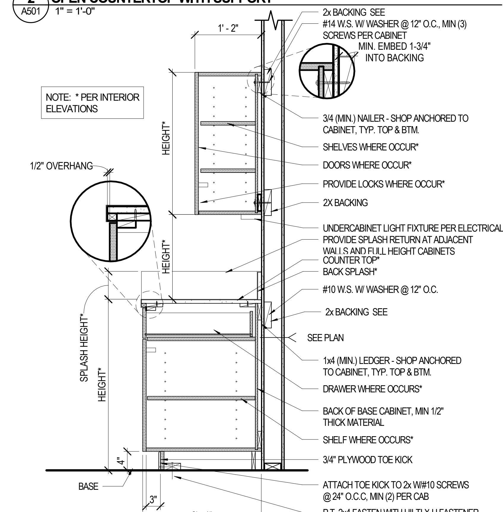
A5 CASEWORK - BASE & UPPER CABINET A501 1" = 1'-0"
