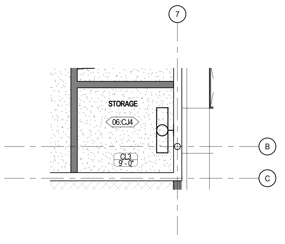
A3 #4 A102 1/4" = 1'-0"
