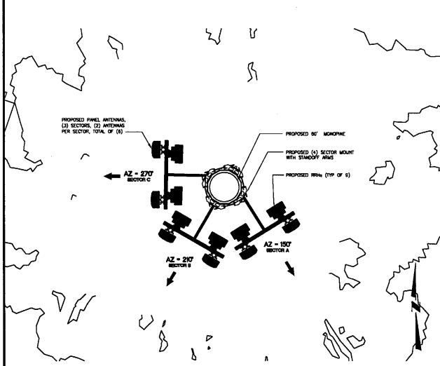
2 ANTENNA LAYOUT SCALE: 3/8" = 1'-0"
