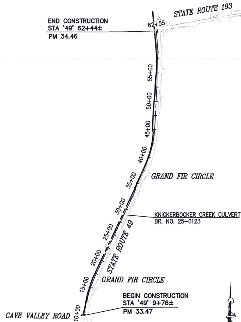
SITE PLAN SCALE: 1" = 500'
