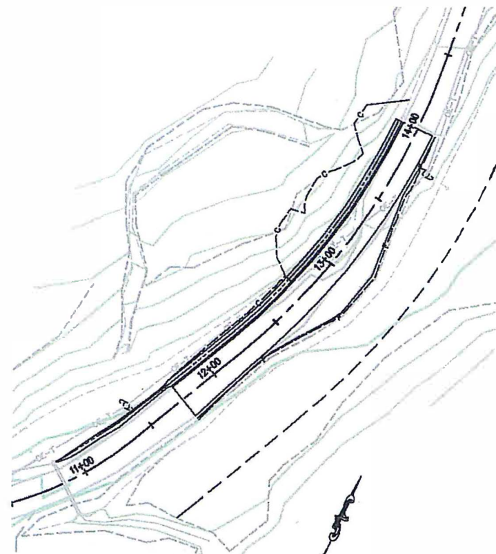
SITE 1 SCALE: 1"=40'
