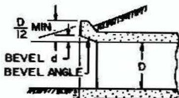
LONGITUDINAL SECTION
