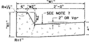
TYPE B2 CURBS See Table A
